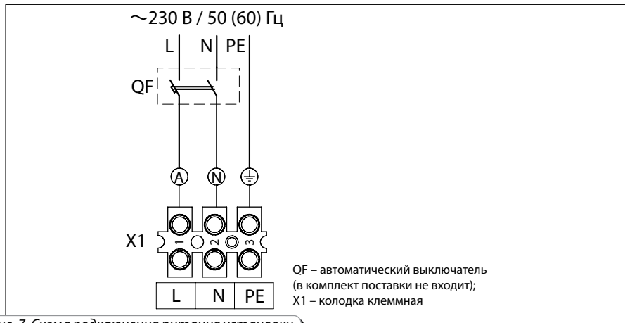
Рис. 7. Схема подключения питания установки
