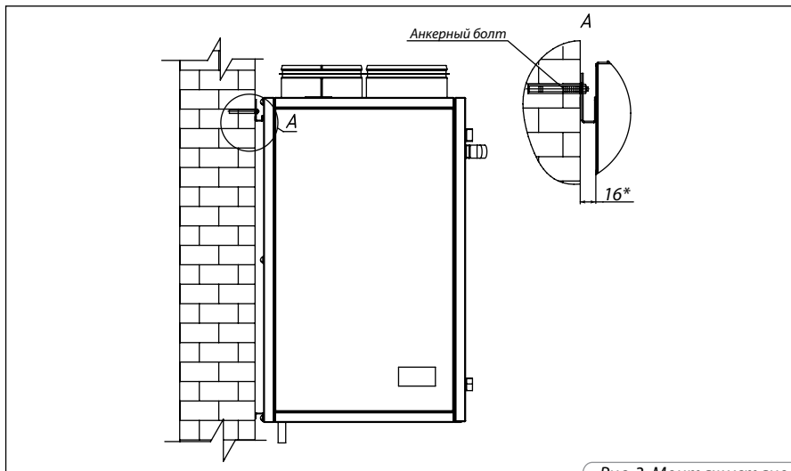
Рис. 3. Монтаж установки
