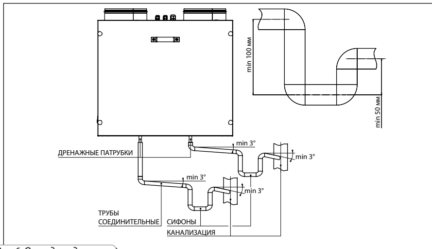
Рис. 6. Отвод конденсата
